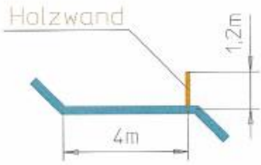
Schnitt A-A
